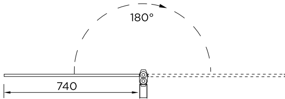
AQ6000 Square Edge Bath Screen
